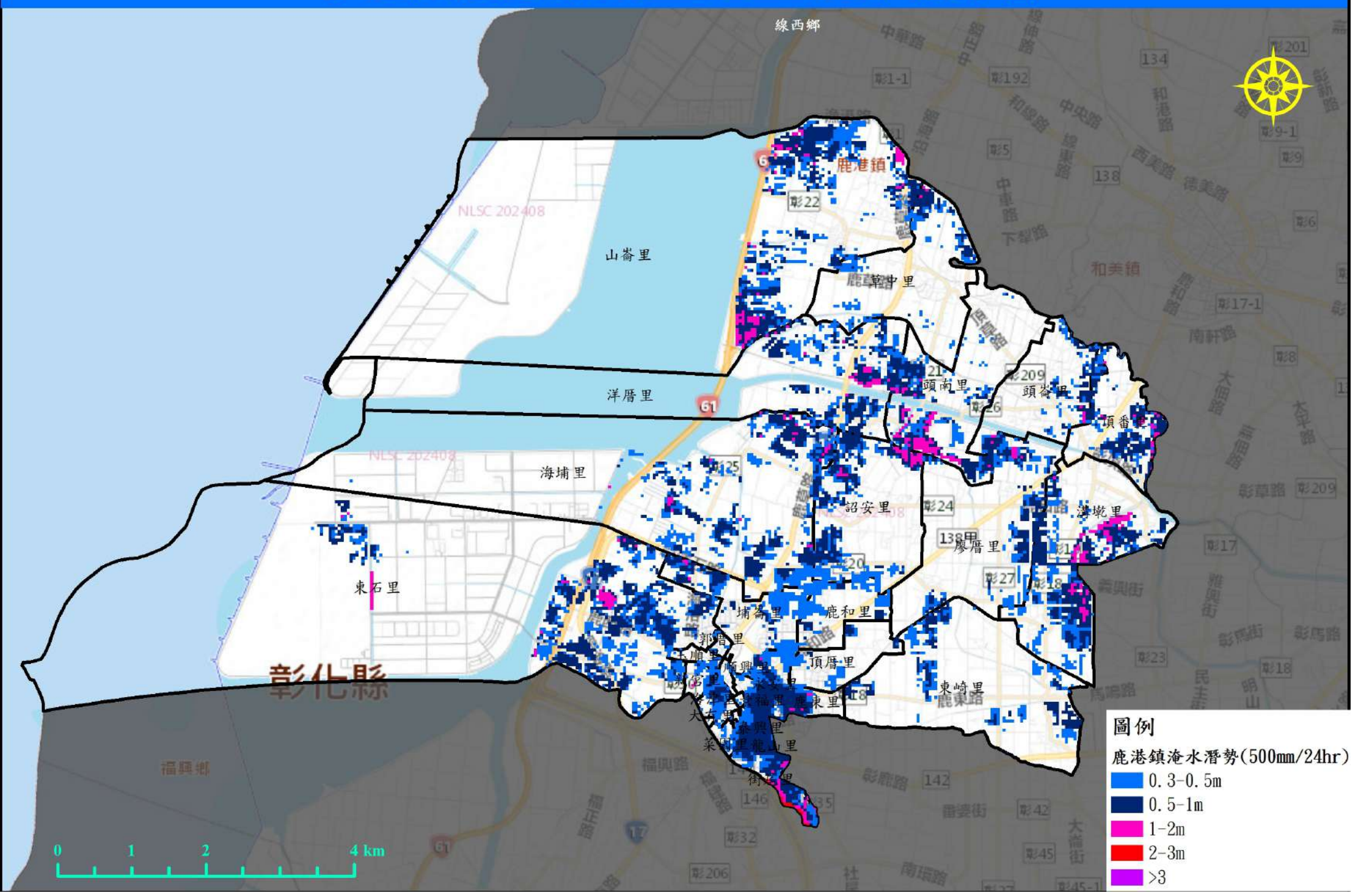
彰化縣鹿港鎮500mm/24hr淹水潛勢圖
